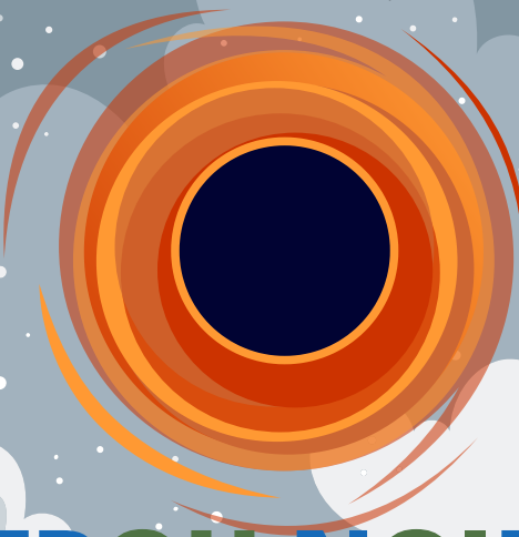
TROU NOIR
