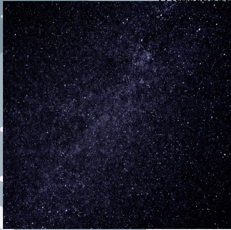
GALAXIE
